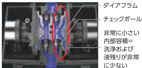
WAGNER DD10 ミドルダイアフラム構造
